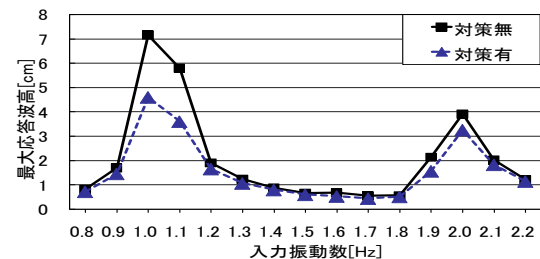
図-2 最大応答波高の比較
