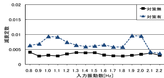
図-3 減衰定数の比較
