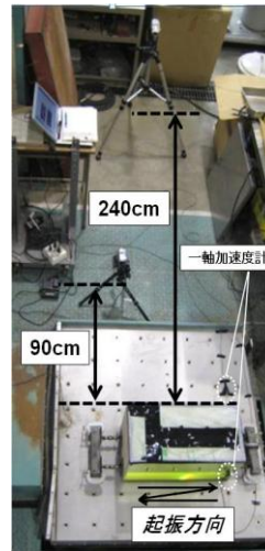
写真-1 実験状況
