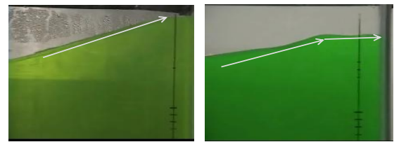
対策無 対策有 写真-3 水槽端部での応答波高 (入力振動数 1.0Hz における静止画)
